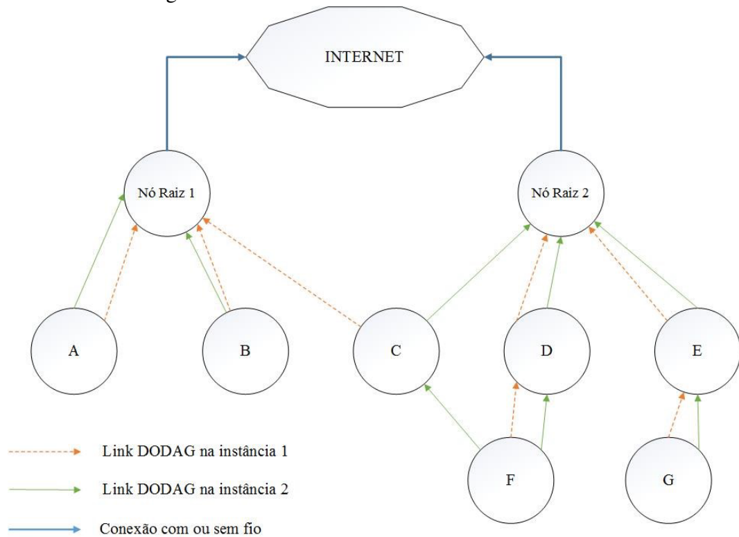
Figura 5 – Rede RPL com 2 DODAGs e 2 instâncias
