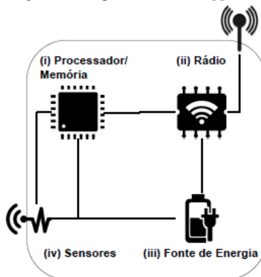
Figura 1 – Arquitetura básica Appliances
