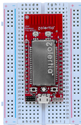
Figura 8 – Zolertia Z1
